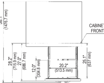
HUR40A-D (TOP VIEW)
