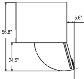
HUF40A (DOOR SWING)
